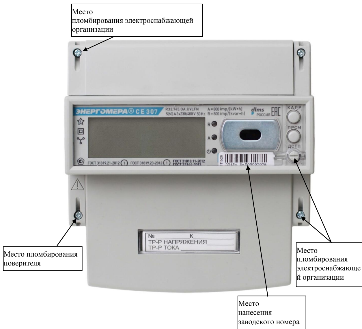
Рисунок 3 – Общий вид счетчика CE307 R33*
